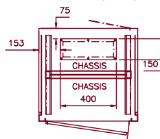
SECTION A-A (OPTION)
